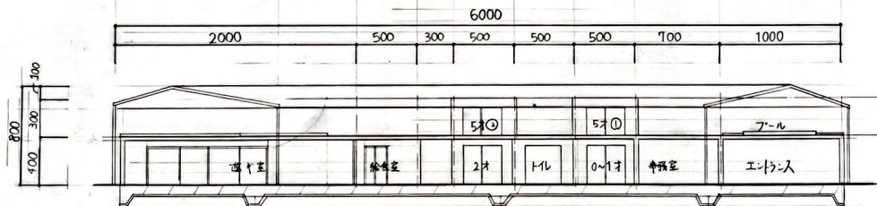
A-A' 断面図
