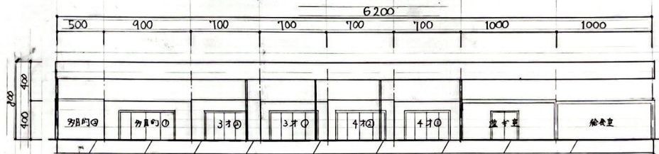
B-B' 断面図
